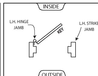
Left Hand Door (Swing In) Left Hand Frame
